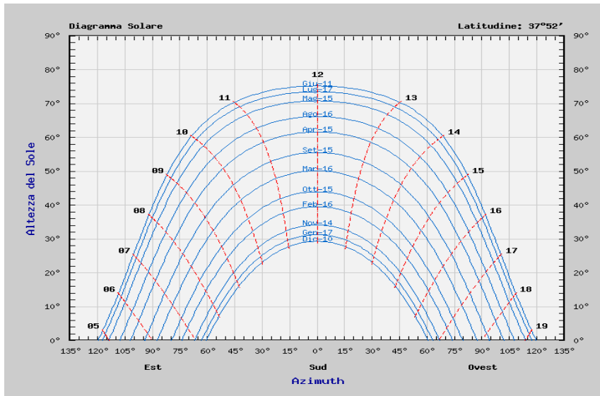
Figura 16. Diagramma solare.
