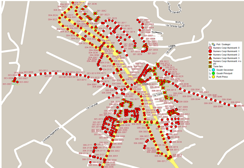
Figura 91. Planimetria Impianto di Pubblica Illuminazione (sezione 1).
