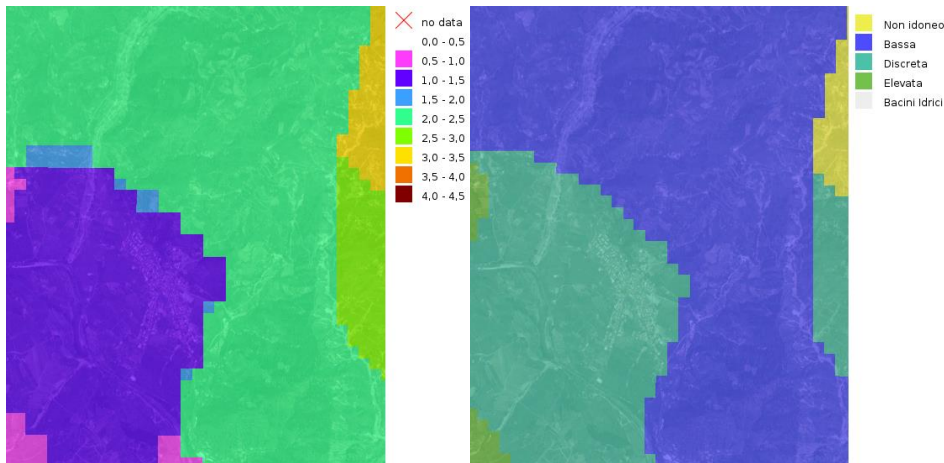
Figura 24. sx) Conducibilità termica calcolata [W/mK]; dx) Idoneità all'utilizzo di sistemi a circuito aperto.
