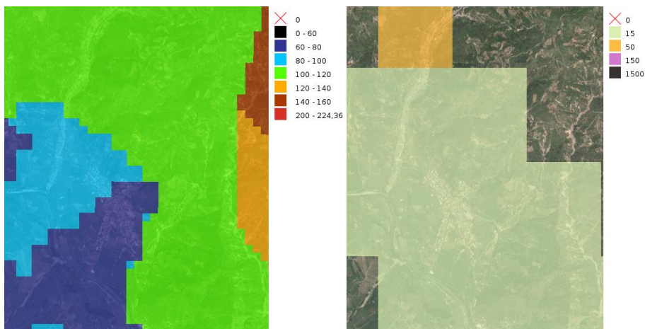
Figura 25. sx) Energia specifica scambiata con il terreno [kWh/m²]; dx) Fabbisogno di calore [TJ/kmq].
